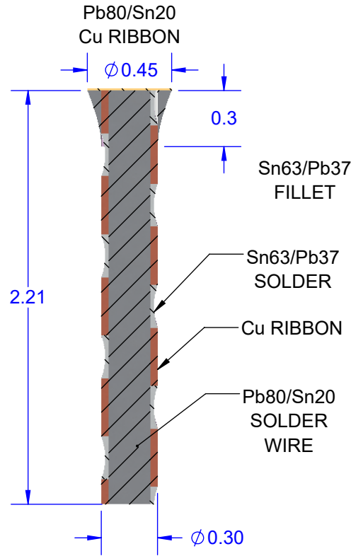
SECTION B-B SCALE 35 : 1
