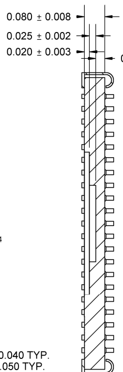
SECTION B-B SCALE 3 : 1.1
