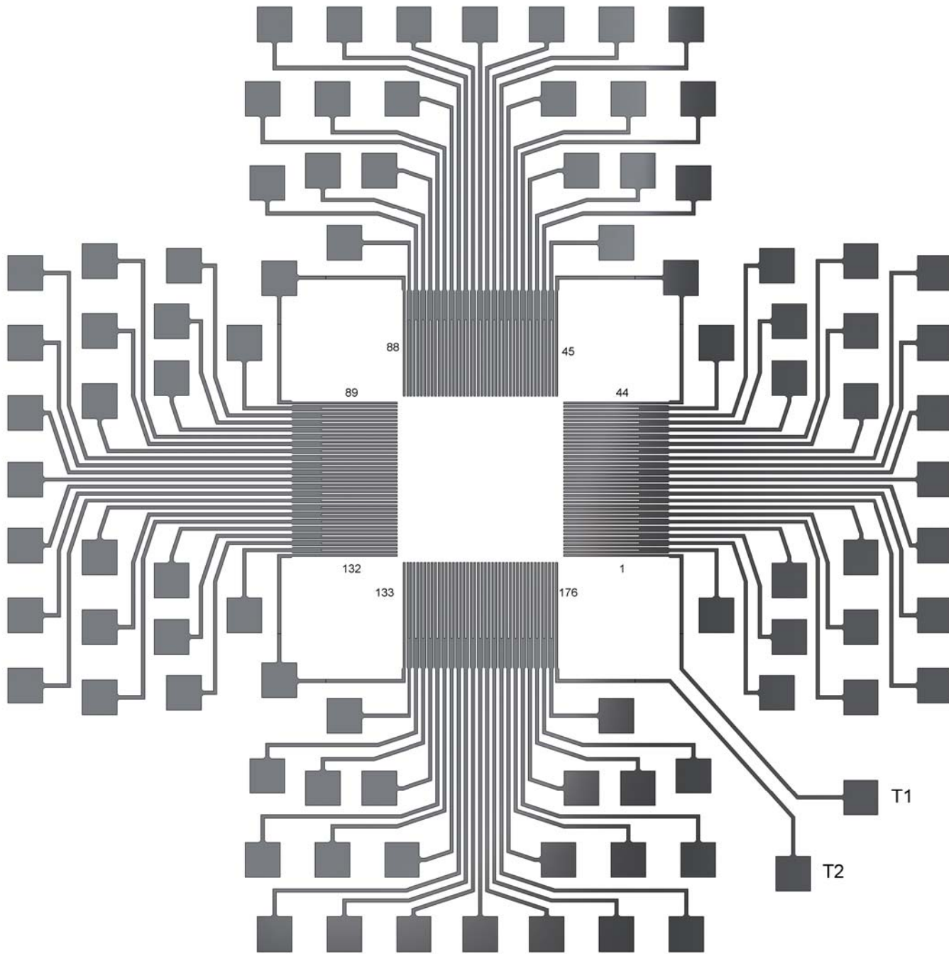
PCB VIEW SCALE: 3.5/1
