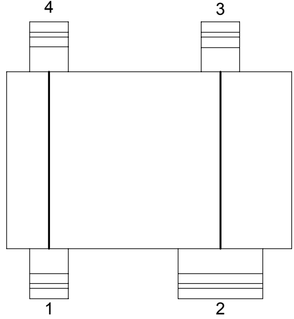
SOT343 - DC1423
