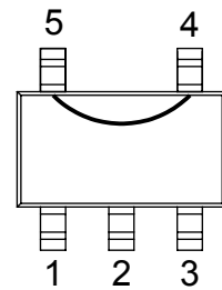
SOT25 - DC45 DWG 120545
