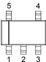
SOT25 - DC51 DWG 120551
