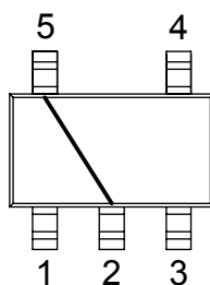
SOT25 - DC52 DWG 120552
