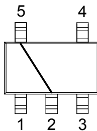
SOT353 - DC52 DWG 120552
