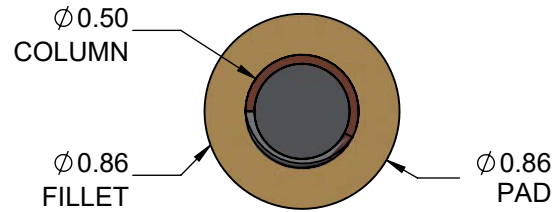
SECTION B-B SCALE 35 : 1
