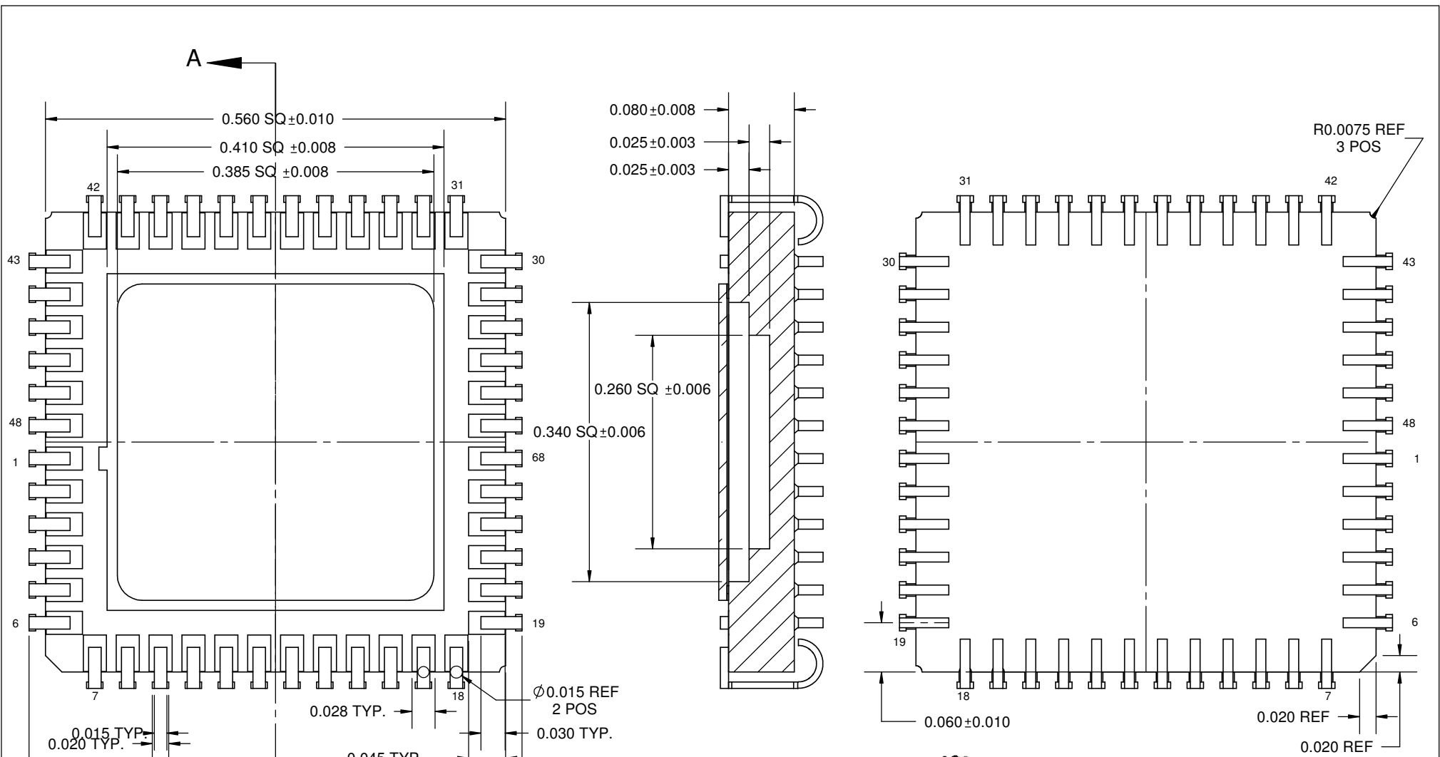
SECTION A-A SCALE 6 : 1
