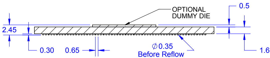
SECTION A-A
